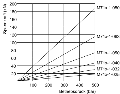
Spannkraftdiagramm Vorhub
