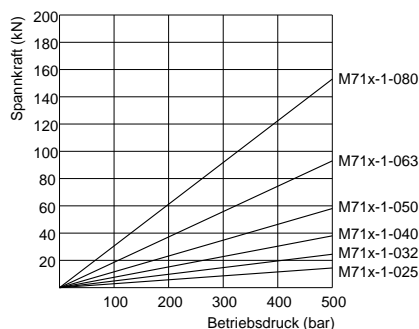
Spannkraftdiagramm Rückhub
